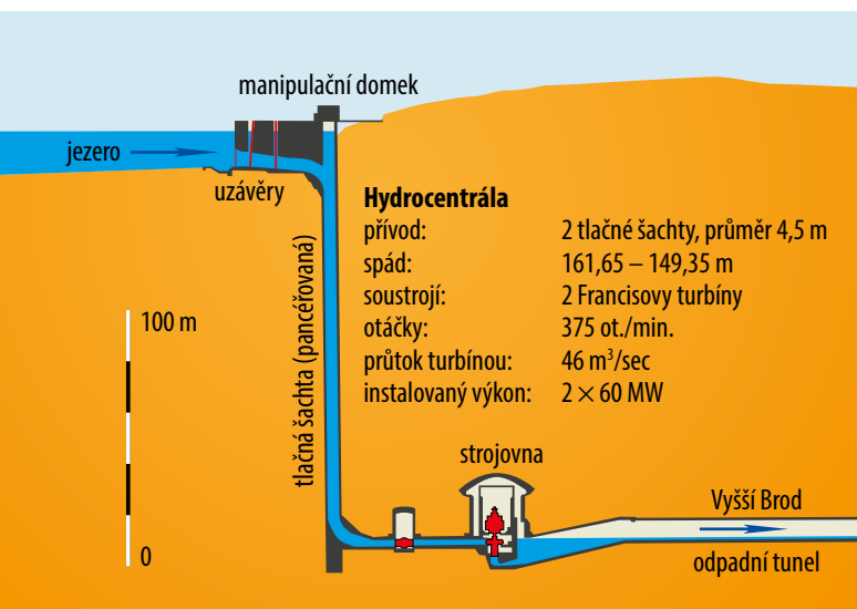
Schéma přehrad s vodní elektrárnou.
